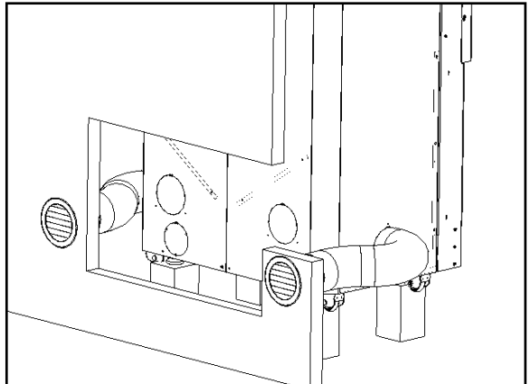
Fig. 7 convezione naturale -
