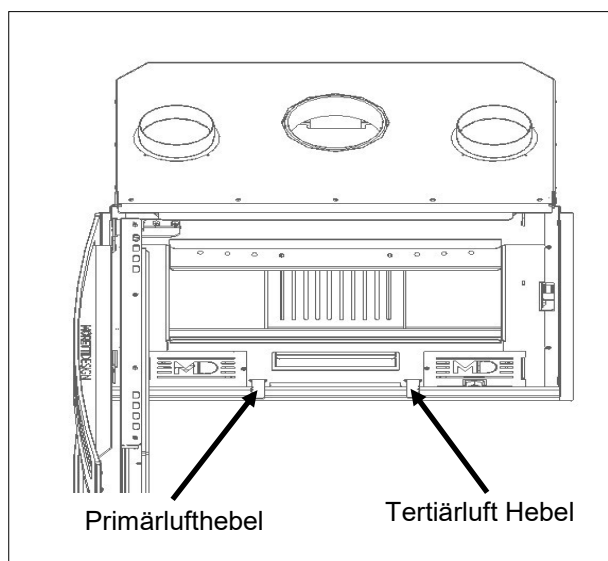
Bild 15: Einstellung der Verbrennungsluft – Slot Wood 7, Slot Wood 8, Slot Wood 9, Slot Flat Wood, Slot Flat Magic
